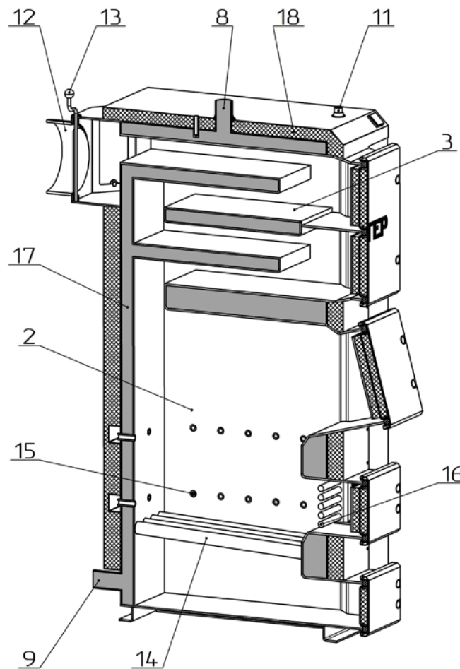
Рисунок 2 – Зовнішній вигляд та основні елементи котла
