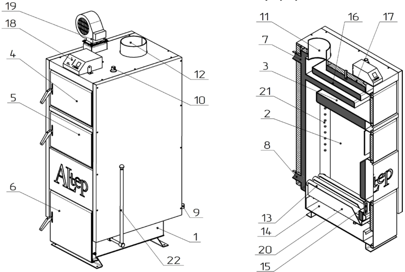
Рисунок 2 – Зовнішній вигляд та основні елементи котла
