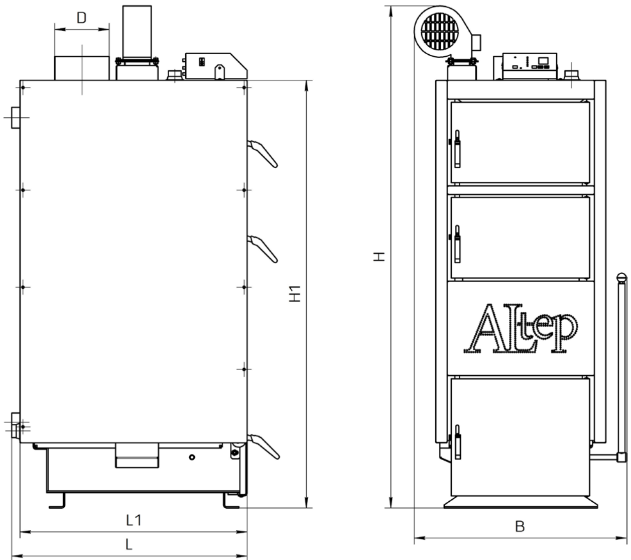
Рисунок 1 – Габаритне креслення котла типу КТ-1-Н
